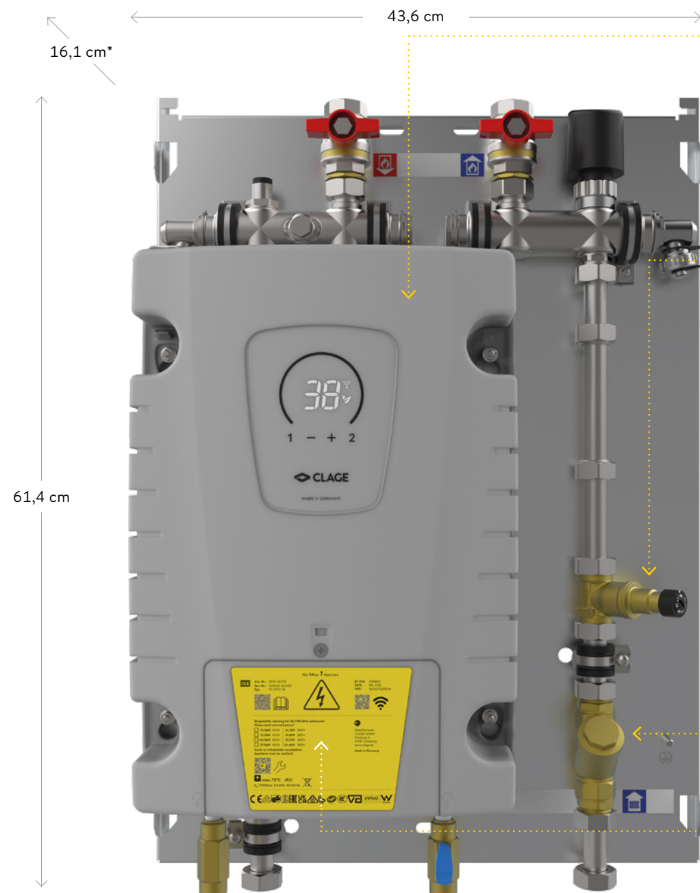
Darstellung einer GTES-E auf Grundblech, ohne Abdeckhaube und Wärmedämmung der Rohrleitung Heizungs-Vorlauf Sekundär
