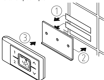
Obrázok A: Montáž s lepiacimi páskami
