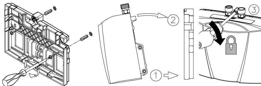
Fig. 5: «Montaje del soporte de pared»
