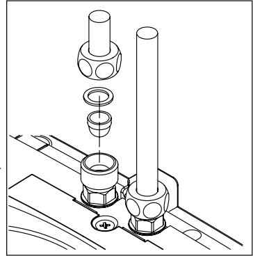
Kuva 11: ”Siivilän vaihtaminen”
