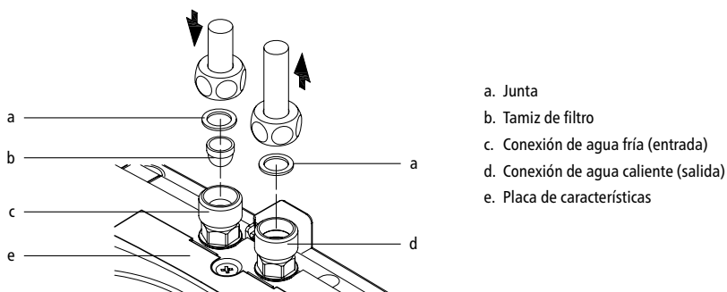
Fig. 6: «Conexión de las tuberías de agua»
