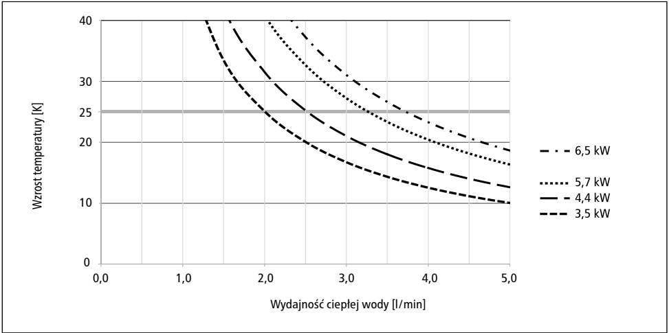
Rys. 10: »Wzrost temperatury i wydajność wody ciepłej«
