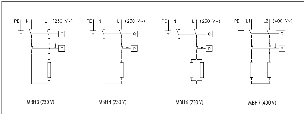
Fig. 7: «Koblingsskjema»
