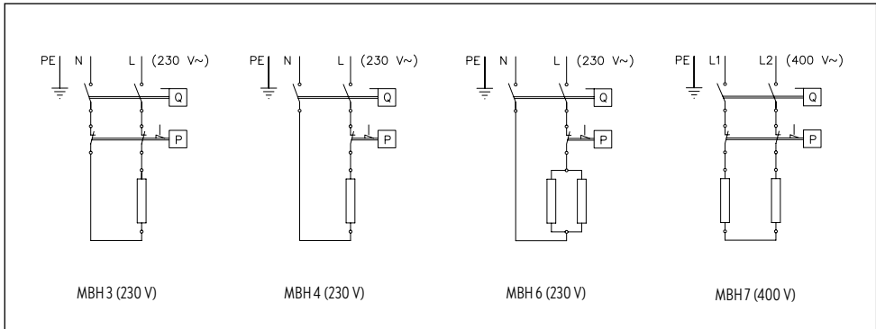
Kuva 7: "Kytentäkaavio"
