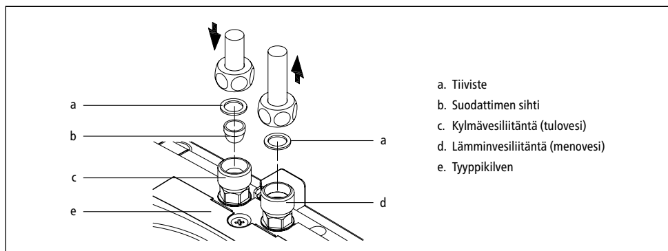
Kuva 6: "Vesijohdojen kytkeminen"
