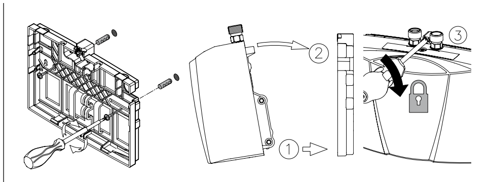
Kuva 5: "Seinäpidikkeen äsennus"
