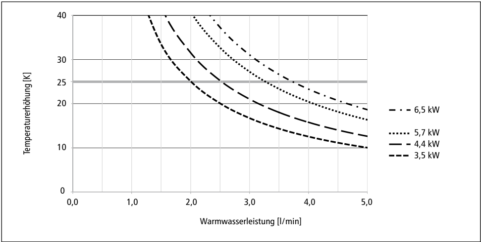
Abb. 10: »Temperaturerhöhung und Warmwasserleistung«
