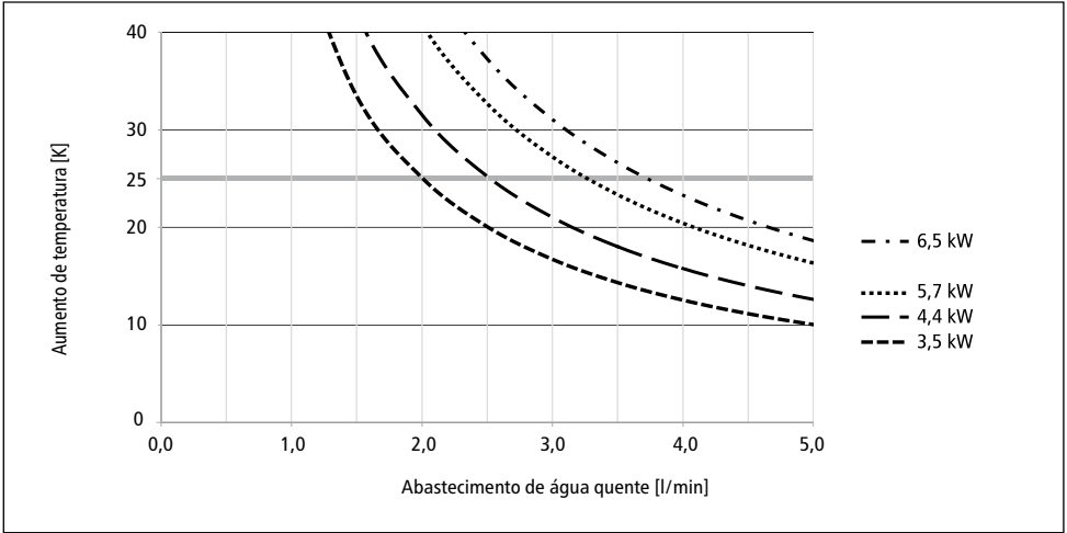
Ilustração 10: »Aumento da temperatura e abastecimento de água quente«
