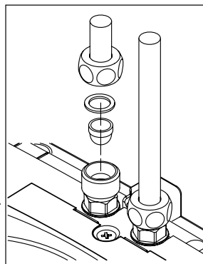
Fig. 11: «Cambio del tamiz de filtro»
