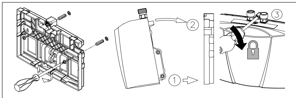
Abb. 5: »Montage des Wandhalters«
